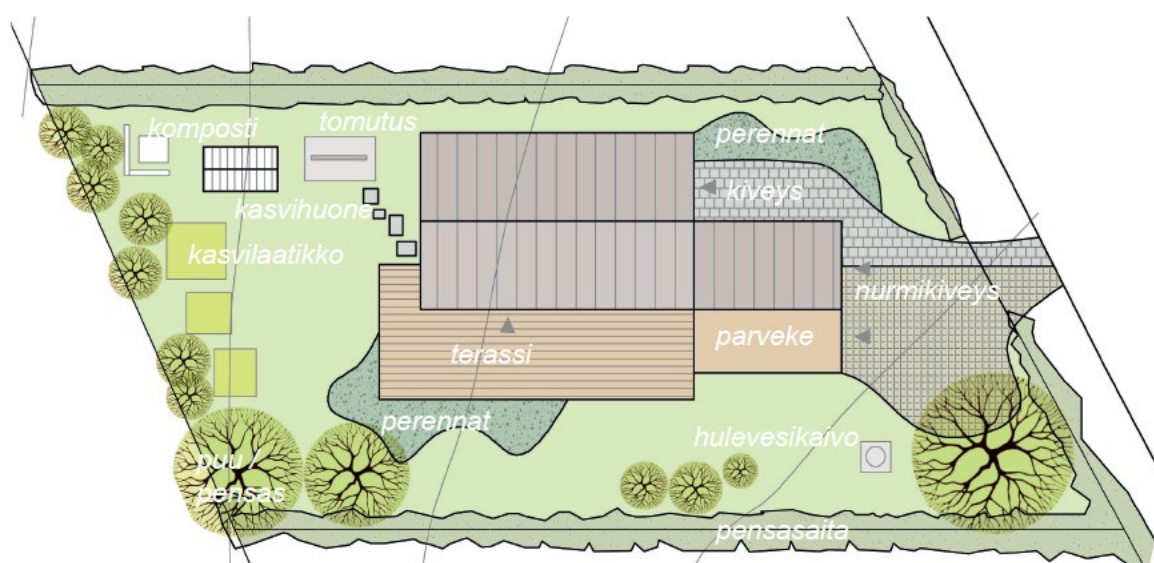
Bild 3. Exempel på en situationsplan som demonstrerar gårdens användning. Parkeringsplatsen har en stenbeläggning med gräs som släpper igenom vatten och ett bärande växtunderlag, som ger näring till gårdsträdet. Regnvatten från taket lagras i dagvattenbrunnen, som finns i gårdens nedre sluttning.
