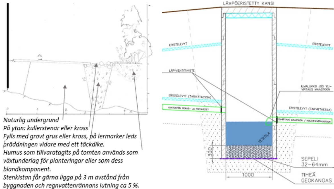
Bild 20. Till vänster: stenkistans yta, förstärkt med kullerstenar. Utdrag ur handboken: Kontrollstrukturer för dagvatten och deras underhåll, Klimatsäker stad, https://www.ilmastotyokalu.fi/sv/ , bild tagen 10.1.2023.
