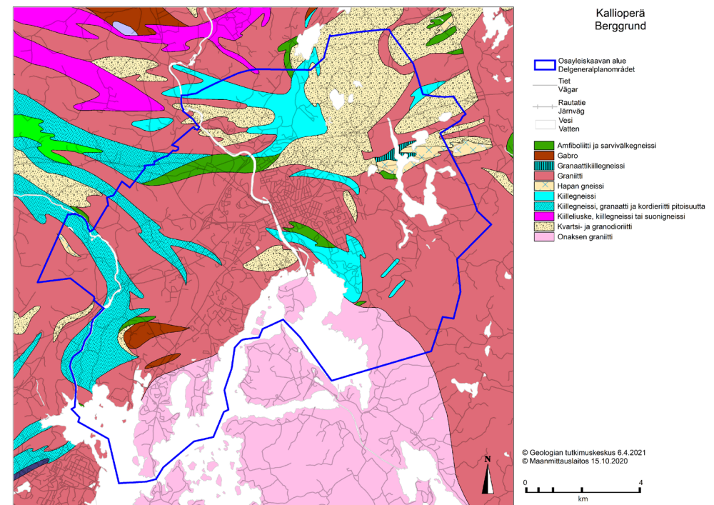
Figur 2: Berggrundskarta.
