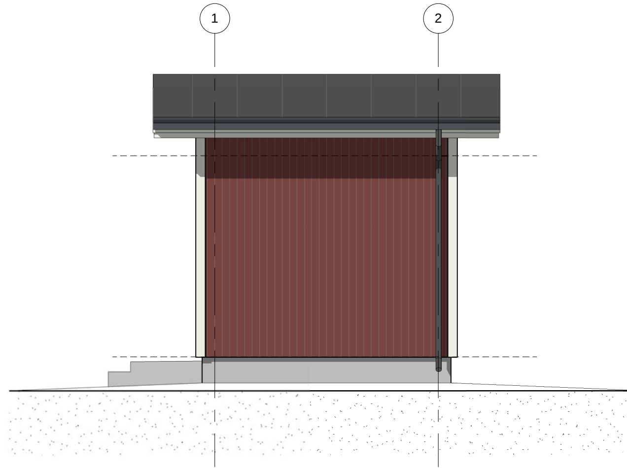
Kaakkoon 1 : 50
