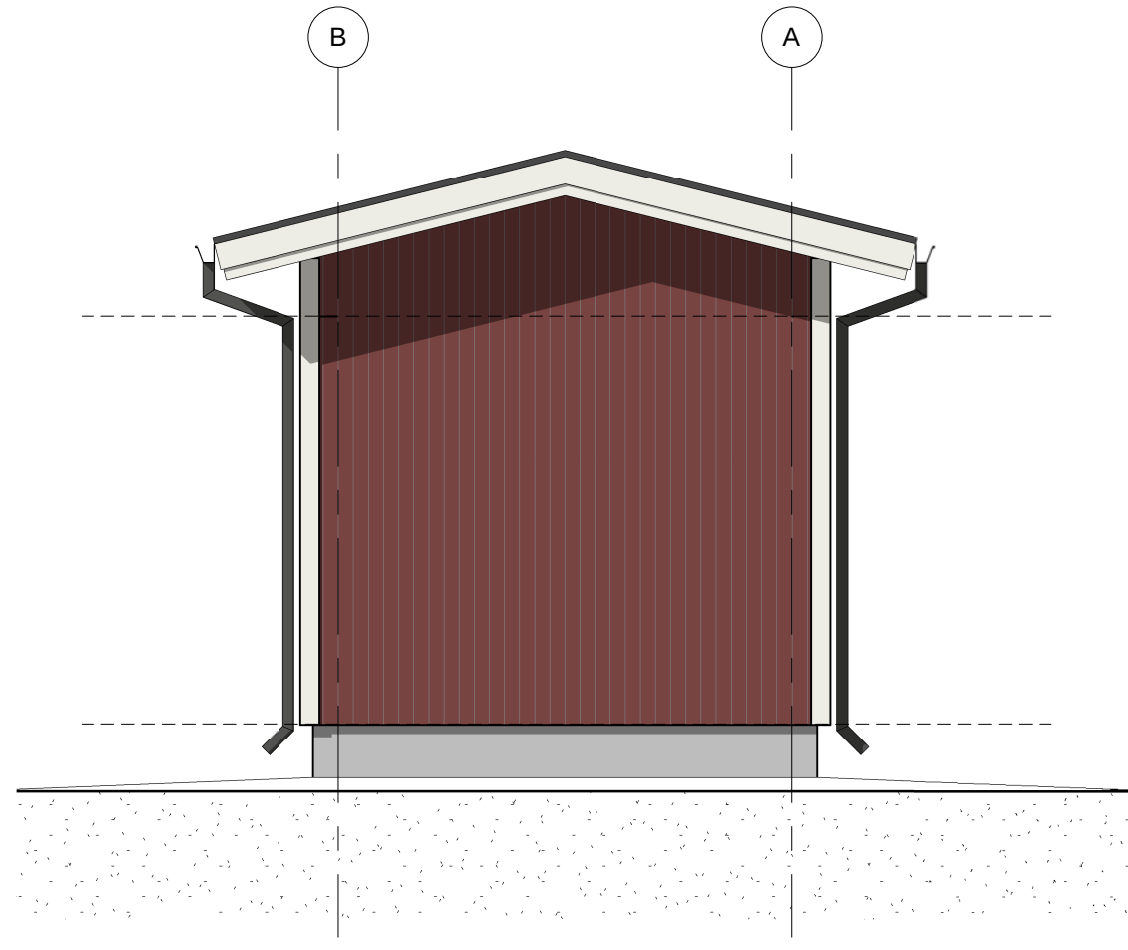
Koilliseen 1 : 50
