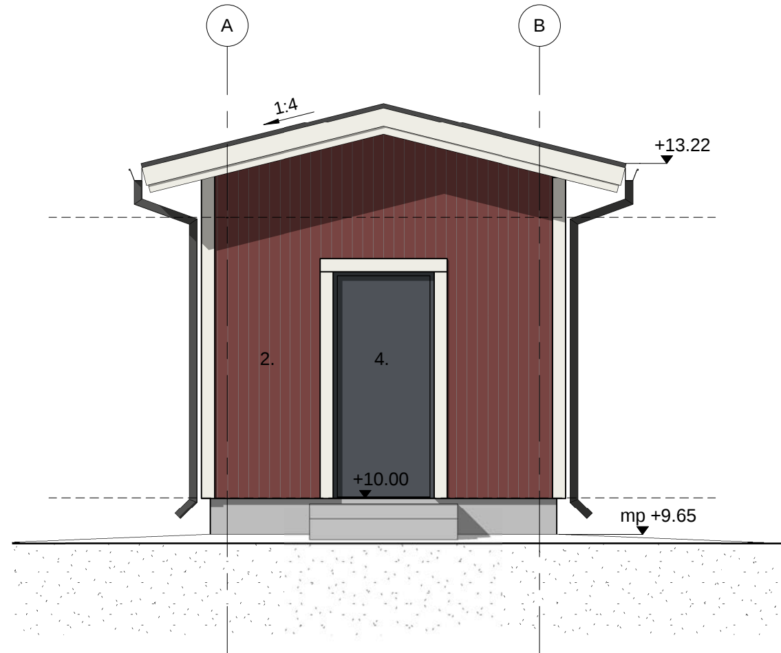
Lounaaseen 1 : 50
