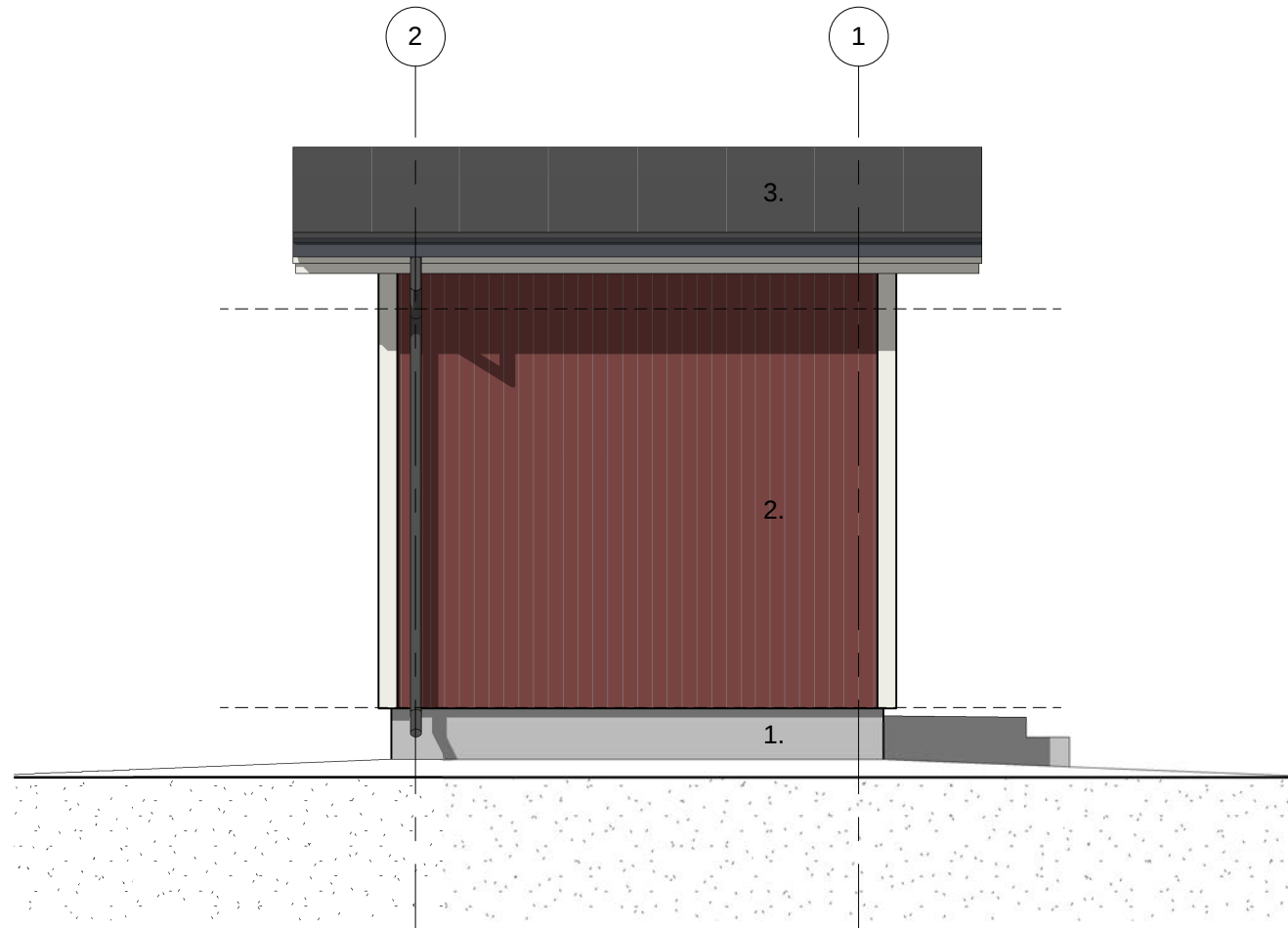
Luoteeseen 1 : 50
